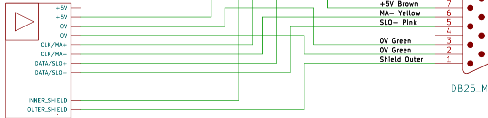
Encoder M2,M4 ENCODER_RL32xxxx
