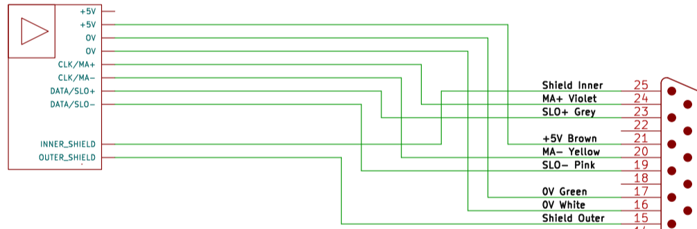
Encoder M1,M2 ENCODER_RL32xxxx
